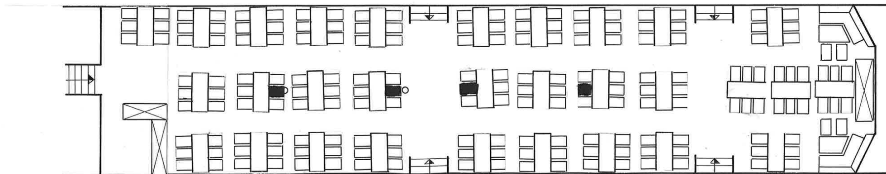
HAUPTDECK 190 PLÄTZE
